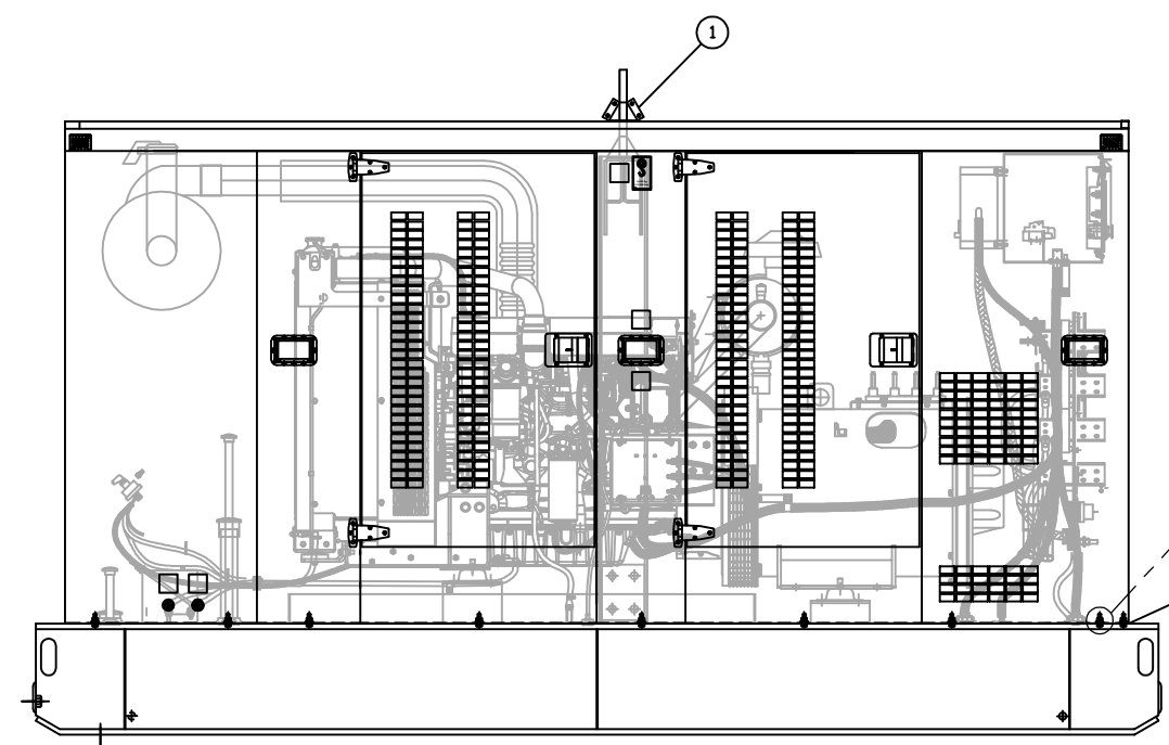
LEFT SIDE
