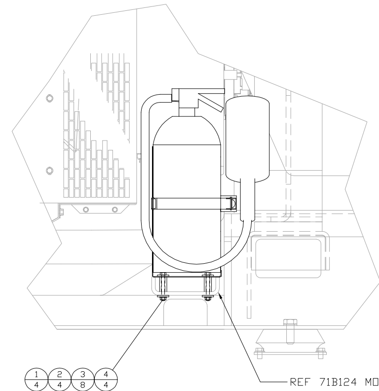
DETAIL A TYP 2 PLACES
